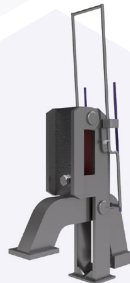
➤ Rochet démontable
